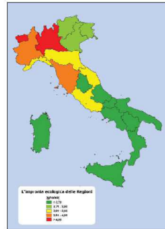
Figura 10: Impronta ecologica delle regioni italiane
